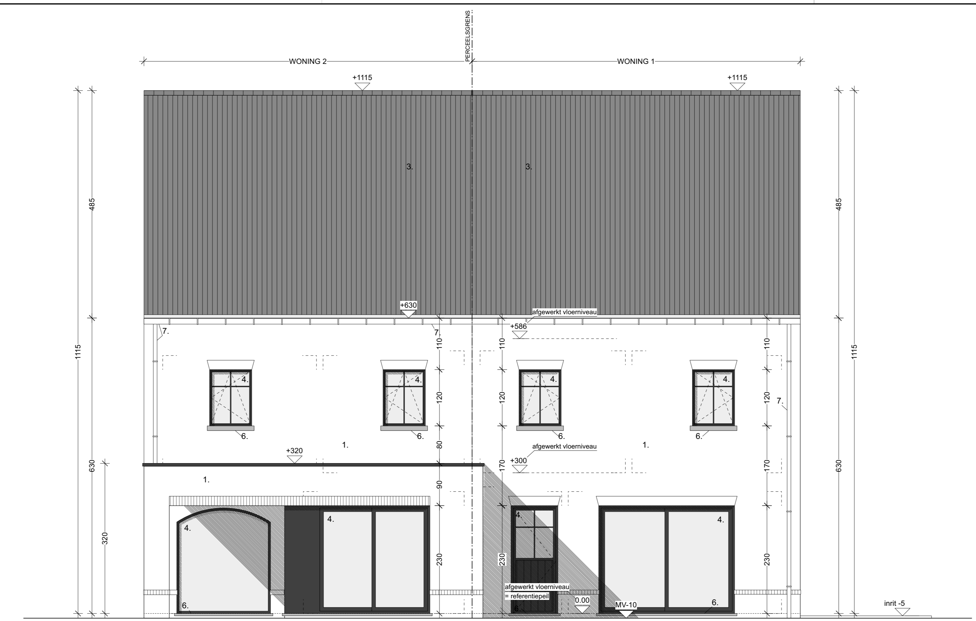
ACHTERGEVEL WONING 1 & 2
