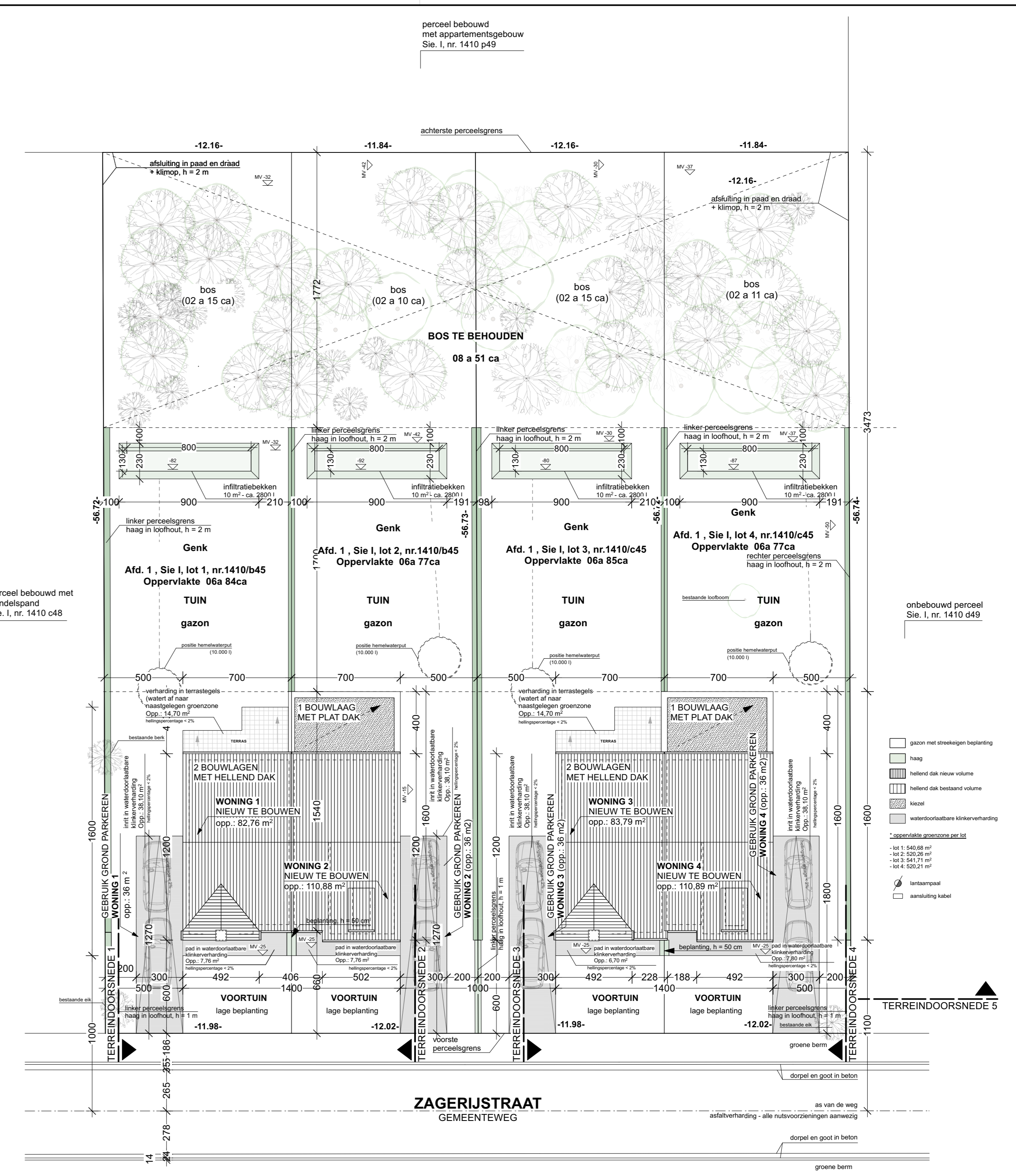
INPLANTINGSPLAN NIEUWE SITUATIE schaal 1/200
