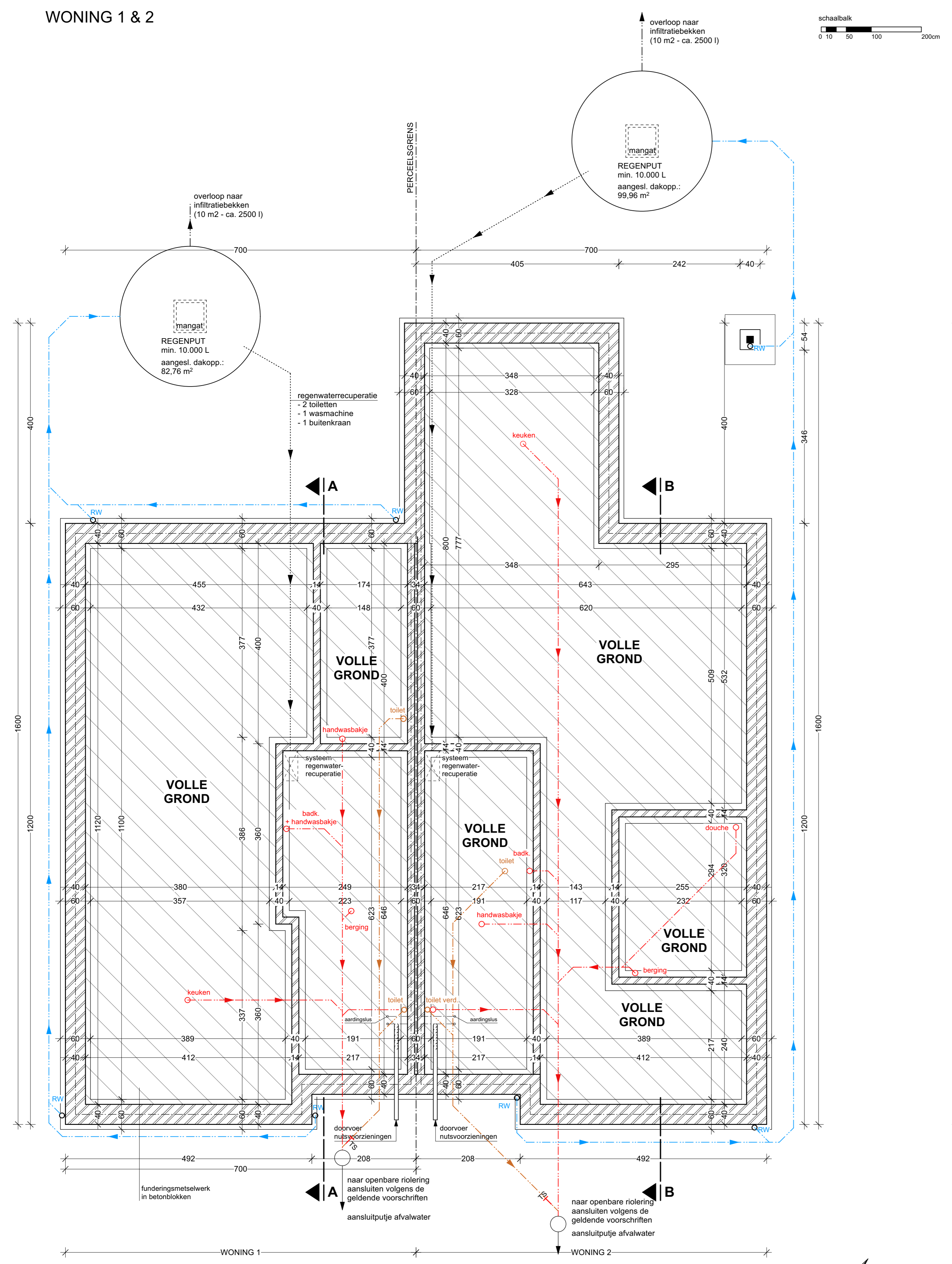
FUNDERINGS- EN RIOLERINGSPLAN WONING 1 & 2
